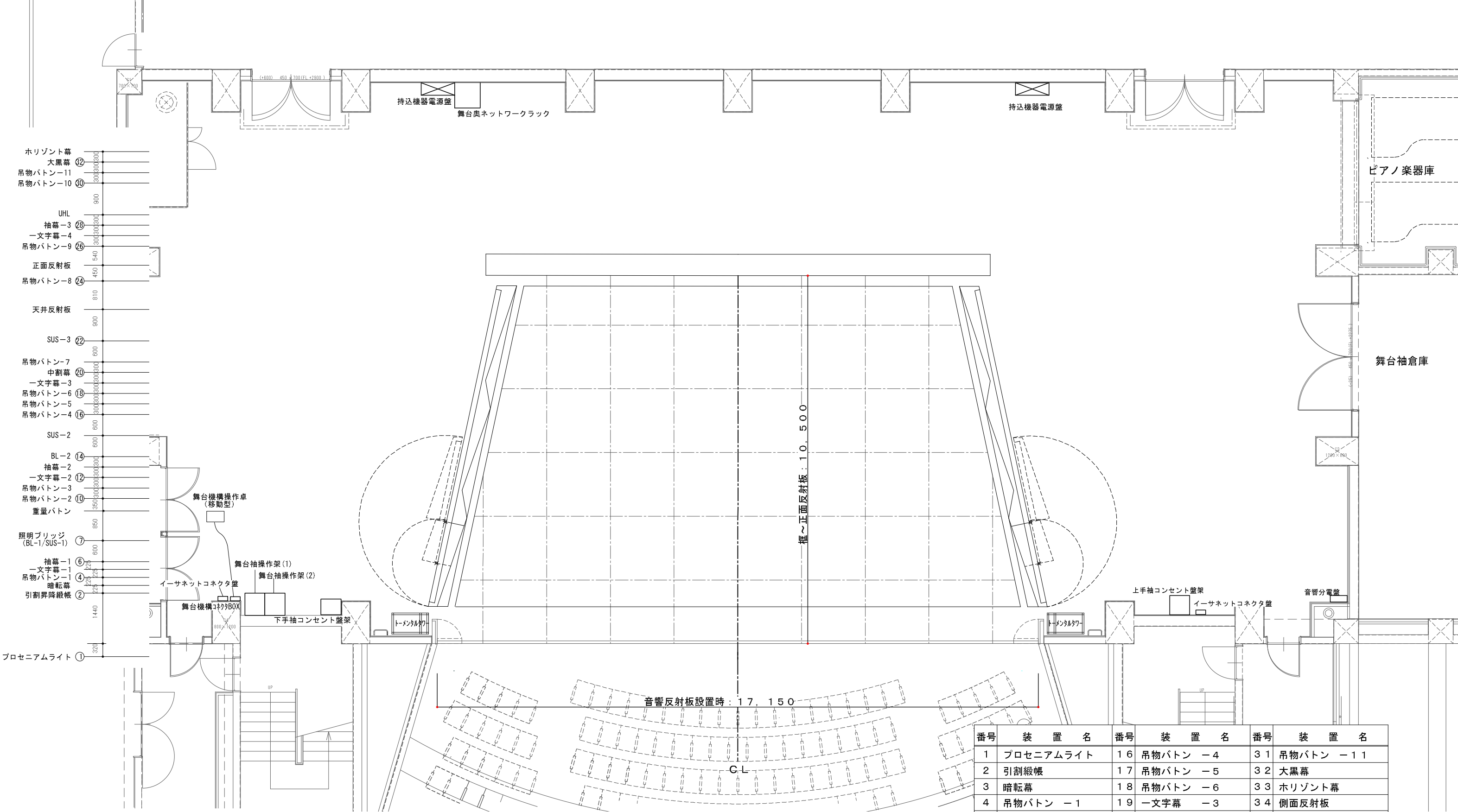
四国中央市市民文化ホール 舞台音響反射板平面図
