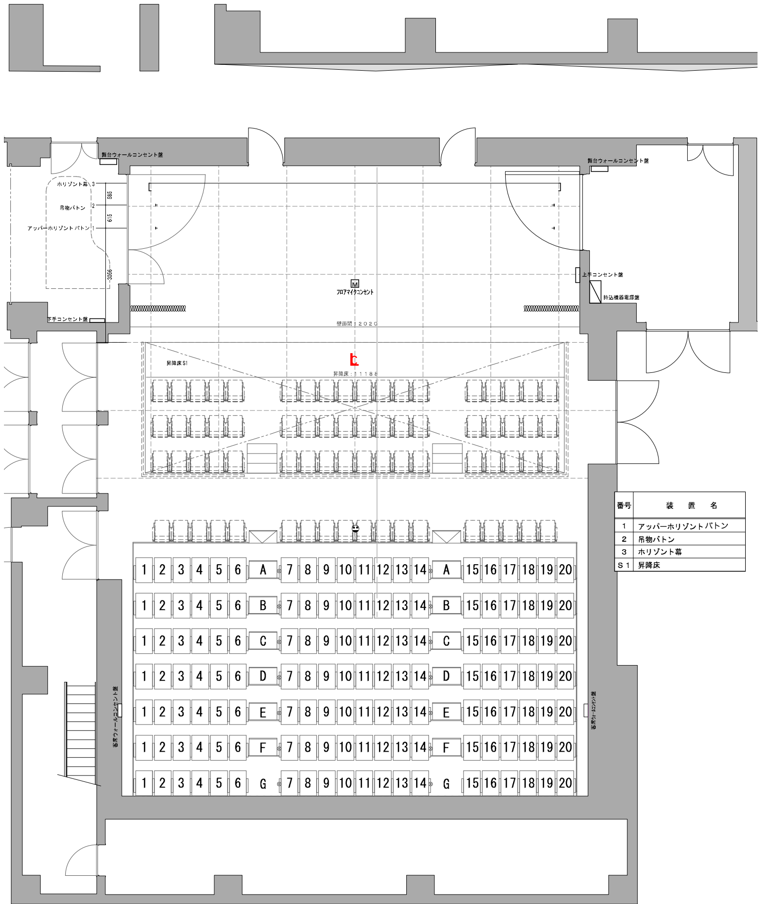
四国中央市民文化ホール 小ホール平面図
